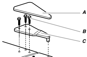
A. Couverture de la charnière supérieure B. Vis de charnière à tête hexagonale de 5/16" C. Charnière supérieure
