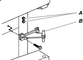
A. Vis de charnière à tête hexagonale de 5/16" B. Charnière centrale
